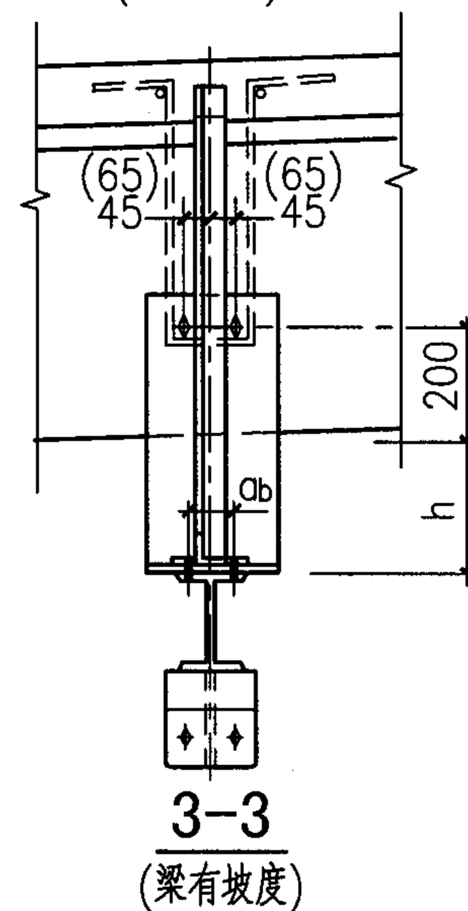
直线轨道与混凝土梁垂直时的连接详图
