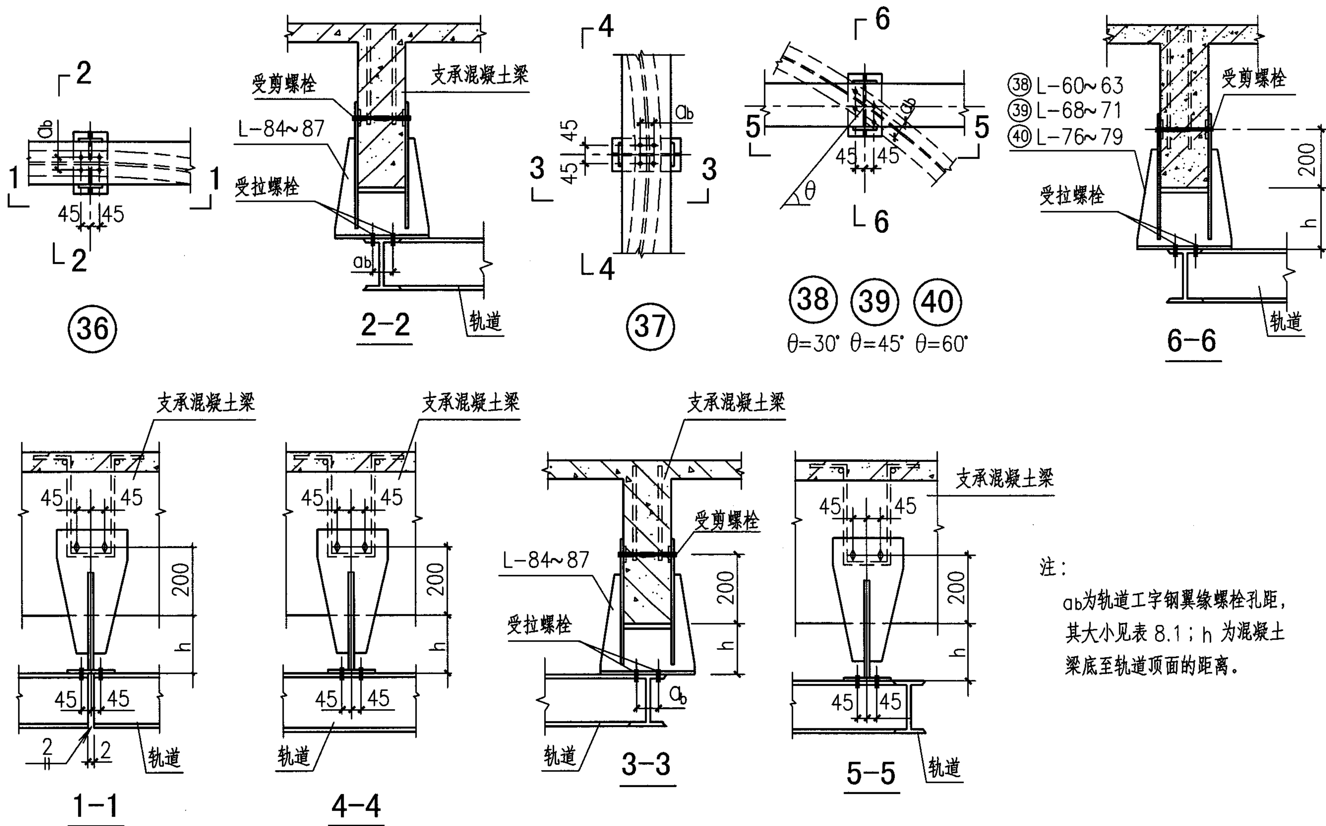
弧线轨道与混凝土梁的连接详图
