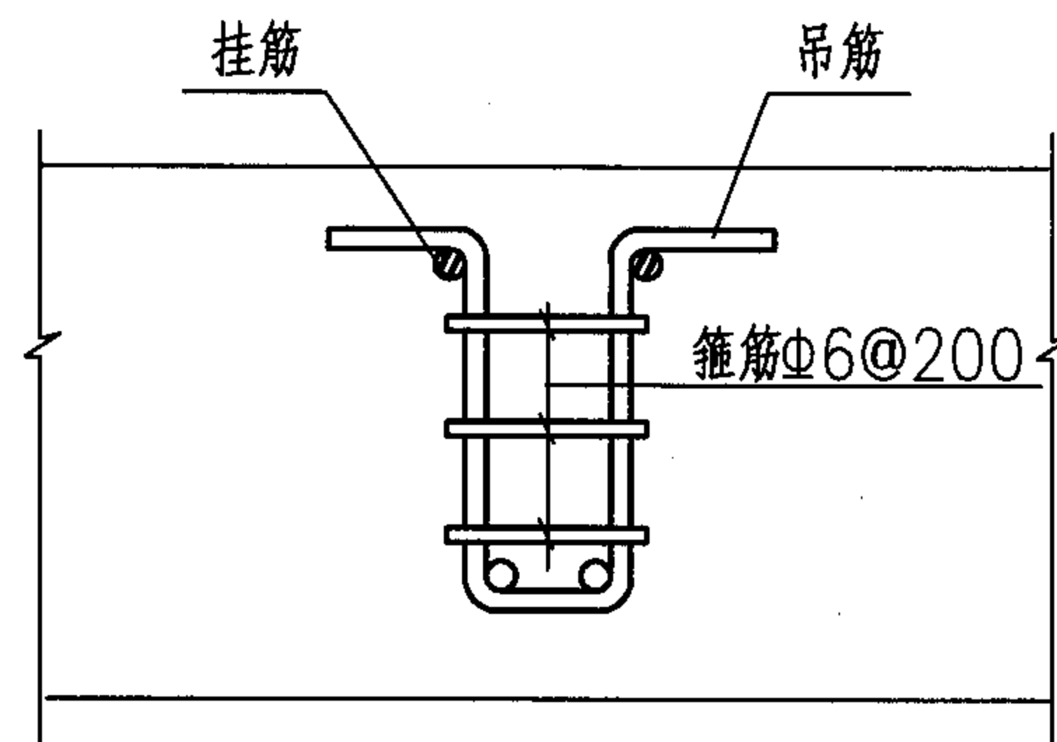
梁内吊筋上应加构造箍筋
