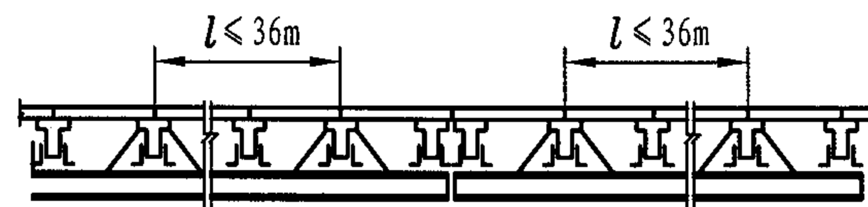
图7.1.2-1 轨道通过变形缝时支撑布置图
