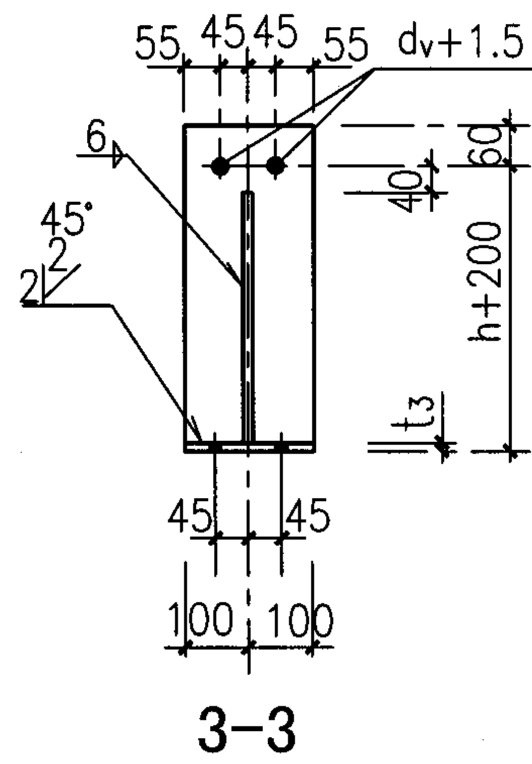
连接件L-84~95详图
