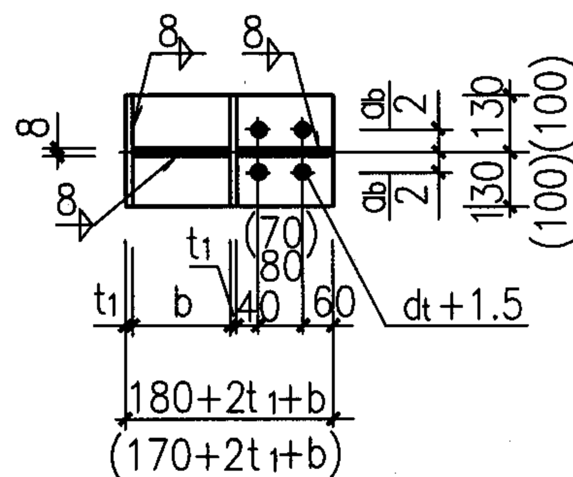
L-56~59选用表
